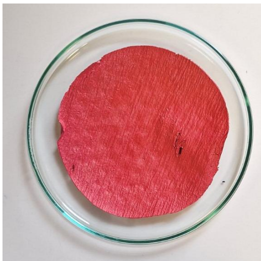
Slika 7.2. Produkt [\text{Ni}(\text{C}_4\text{H}_7\text{O}_2\text{N}_2)_2]
