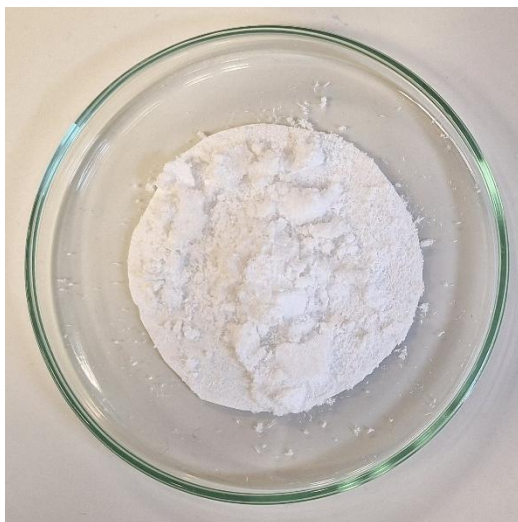
Slika 11.1. Produkt K_3[Al(C_2O_4)_3] \cdot 3H_2O
