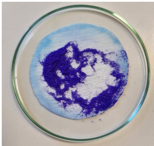
Slika 7.1. Produkt [\text{Ni}(\text{NH}_3)_6]\text{Cl}_2
