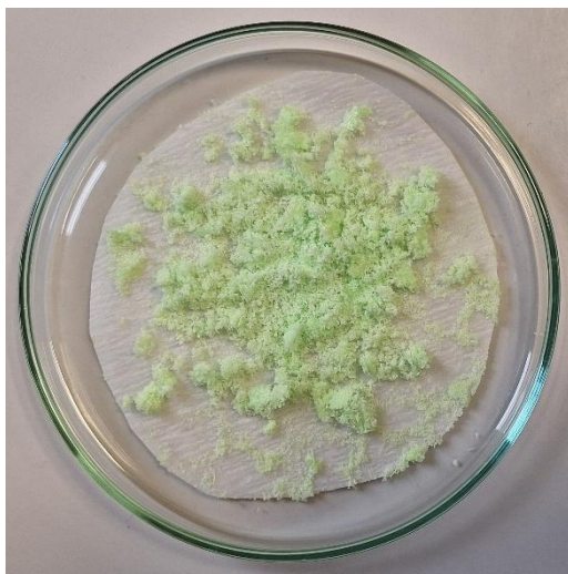
Slika 10.1. Produkt K_3[Fe(C_2O_4)_3] \cdot 3H_2O
