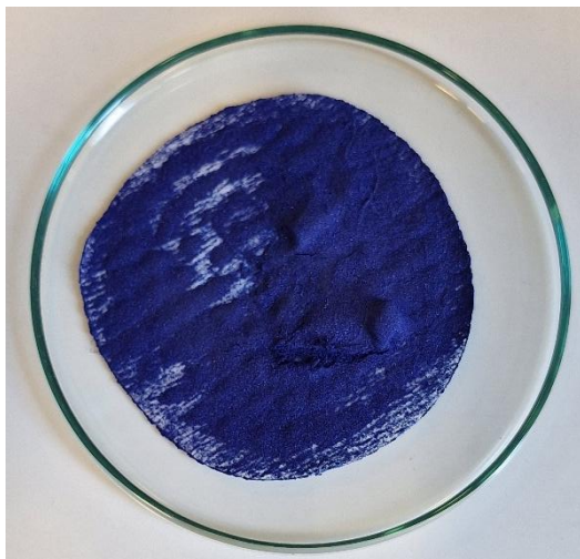
Slika 6.1. Produkt \text{Hg}[\text{Co}(\text{NCS})_4]
