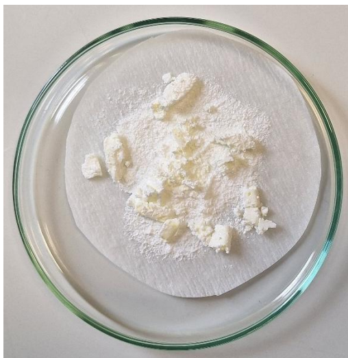
Slika 3.1. Produkt [\text{Cu}(\text{SC}(\text{NH}_2)_2)_3]_2\text{SO}_4 \cdot \text{H}_2\text{O}
