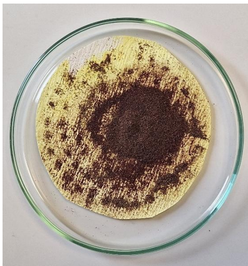
Slika 1.1. Produkt K_3[Cr(O_2)_4]
