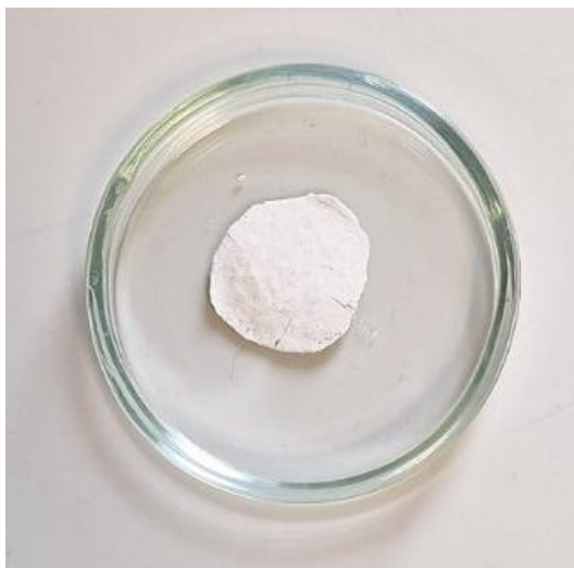
Slika 1.2. Produkt KB(C_6H_5)_4
