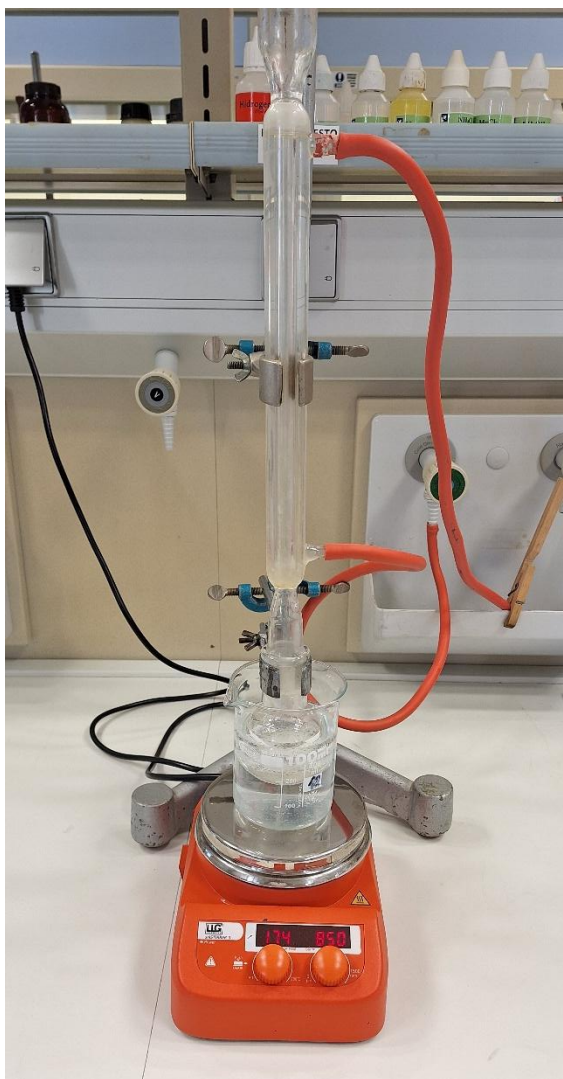
Slika 11.2. Aparatura za izvođenje sinteze kompleksa K_3[Al(C_2O_4)_3] \cdot 3H_2O
